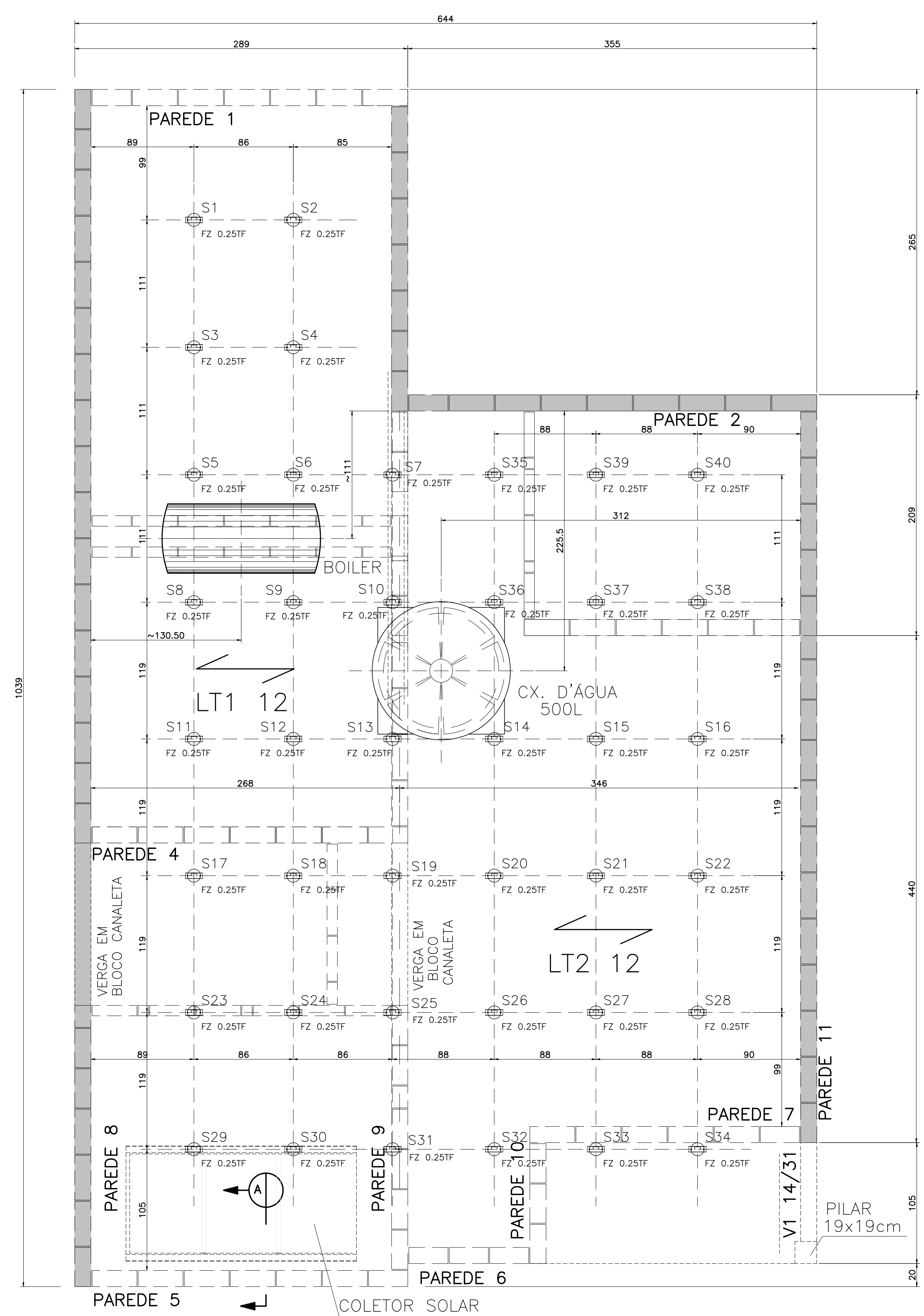
COBERTURA-FORMAS LAJE PRÉ-MOLDADA E LOCAÇÃO DOS EQUIPAMENTOS 2 DORMITÓRIOS ESC. 1:25
