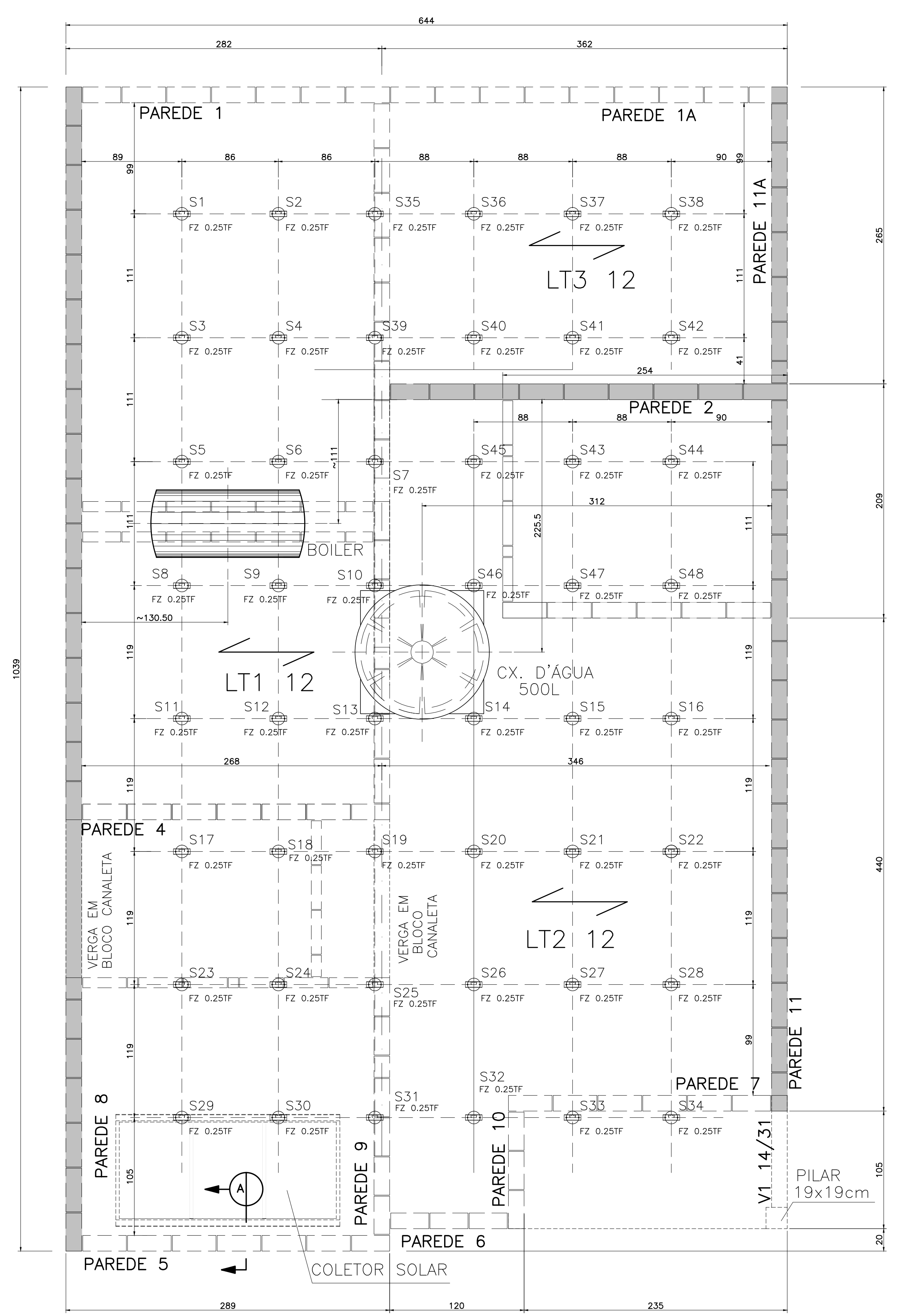
COBERTURA-FORMAS LAJE PRÉ-MOLDADA E LOCAÇÃO DOS EQUIPAMENTOS 3 DORMITÓRIOS ESC. 1:25
